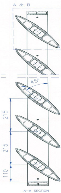
A-A SECTION
